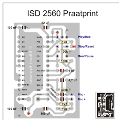
Schema praatprint
